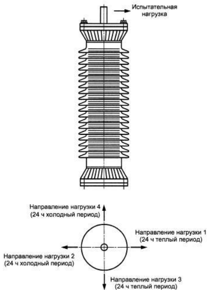
Рисунок 4 - Термомеханические испытания
