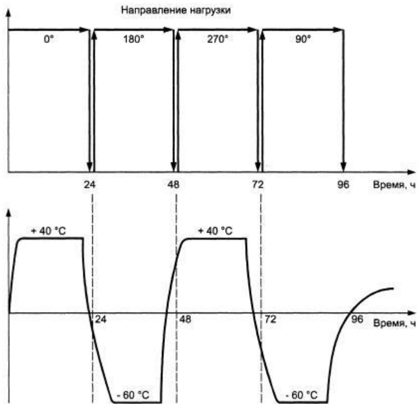
Рисунок 4 - Термомеханические испытания
